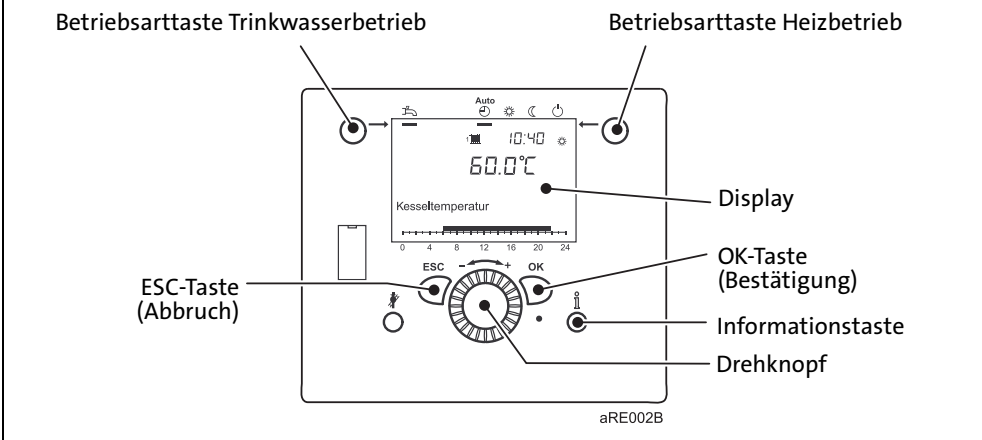
Abb 1: Bedienelemente
